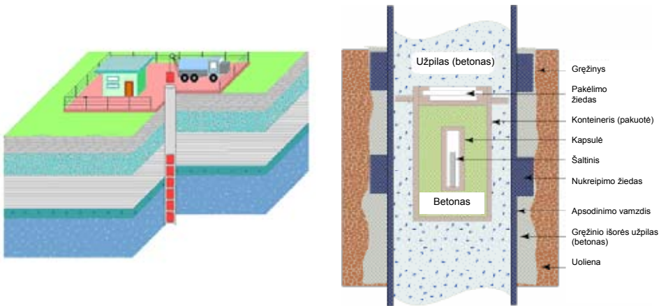
6. Pav. Panaudotų uždarytų šaltinių laidojimas „BOSS“ sistemos gręžinyje: pakuotės su panaudotais šaltiniais ir artimosios aplinkos komponentai [17]
