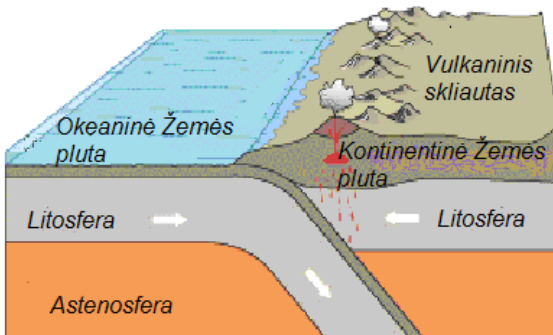
9 pav. Subdukcijos zonos susidarymas [27]
