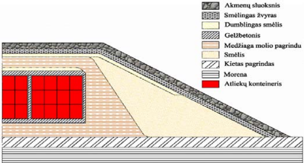
5 pav. Uždaryto „piliakalnio“ pavidalo kapinyno su inžineriniais barjeriais skersinis pjūvis [13]
